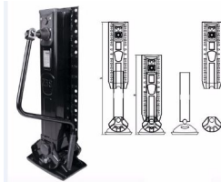
Produkt Anhängerparkfuss
