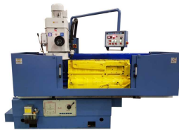
Produkt Flachsleifmaschine
