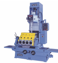
Produkt Motor-Regenerationsmaschine
