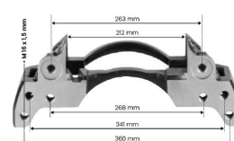
Продукт. Скоба Суппортпа
