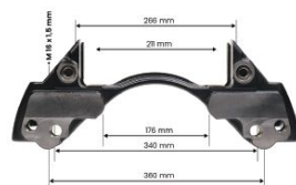
Продукт. Скоба Суппорта
