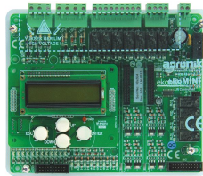
Ürün Asansör Kumandaları Ve Panelleri
