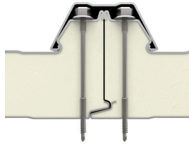
Ürün Solar Uyumlu 4 Hadveli Kepli Çatı Paneli
