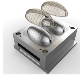
Ürün Plastik Enjeksiyon Kalıbı
